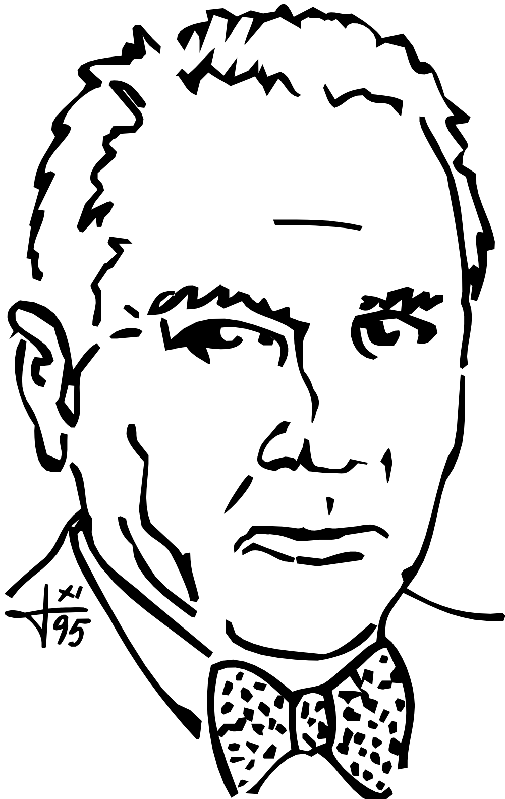
Millikan
