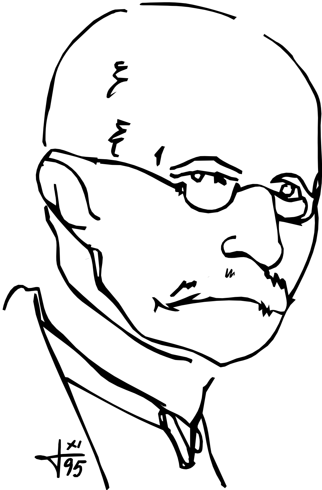
Planck
